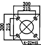
DISTANCIA ENTRE PERNOS PARA ALTURAS: 3M-3,5M-4M-5M-6MTS.
