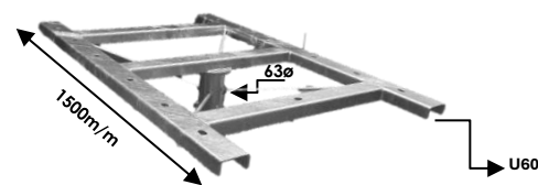
CRUCETA RECTANGULAR 6-8 PROYECTORES
