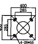
DISTANCIA ENTRE PERNOS PARA ALTURAS: 7MTS-8MTS-9MTS.
