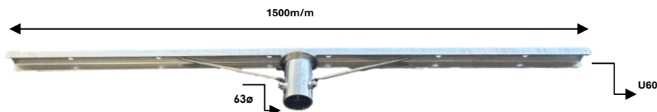
CRUCETA 3-4 PROYECTORES
