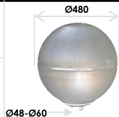
ESFERA PRISMATICA DE 480Ø Y MATERIAL POLICARBONATO ANTIVANDALICO. REF:GP-48PL
